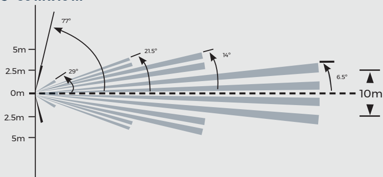
VUE DU DESSUS - 50 m x 10 m
