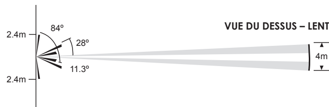
VUE DU DESSUS – LENTILLE 40 m x 8 m
